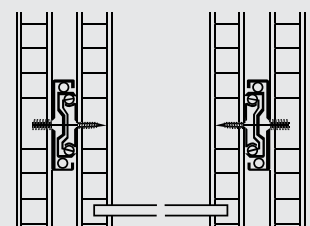
Side Mounted ติดตั้งแบบรับข้าง
