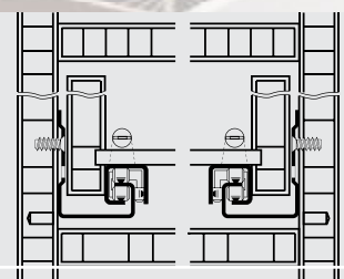
Concealed Mounting ติดตั้งแบบซ่อน
