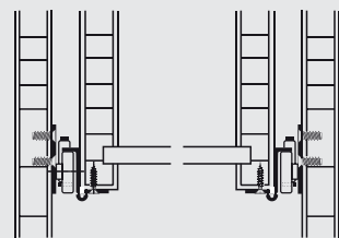
Bottom Mounted ติดตั้งแบบรับได้
